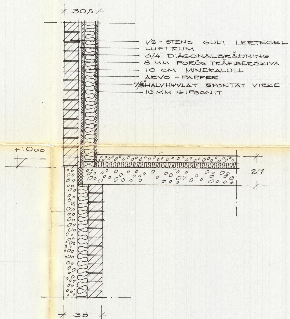
SEKTION GENOM GAVELVÄGG
