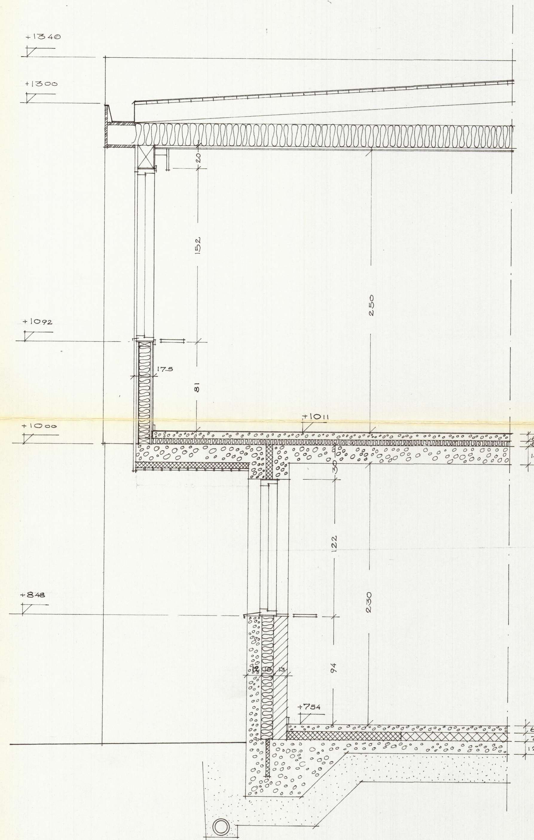
SEKTION VID VETERINÄRS LABORATORIUM — KANALI
