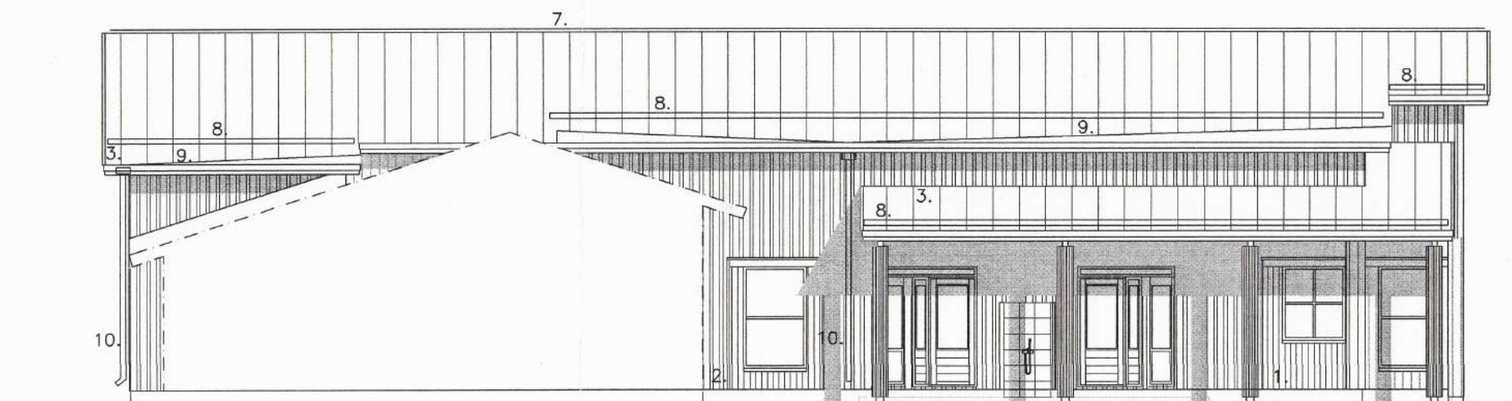
FASAD MOT SYD SKALA 1/100
